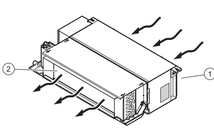
1 Luchtaanzuiging 2 Luchtverdeling
