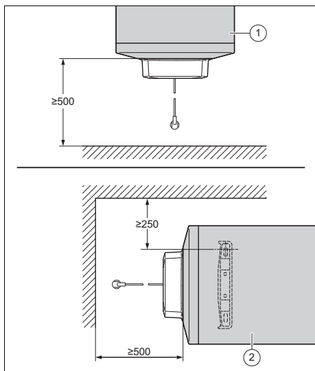
1 Posición de montaje vertical
